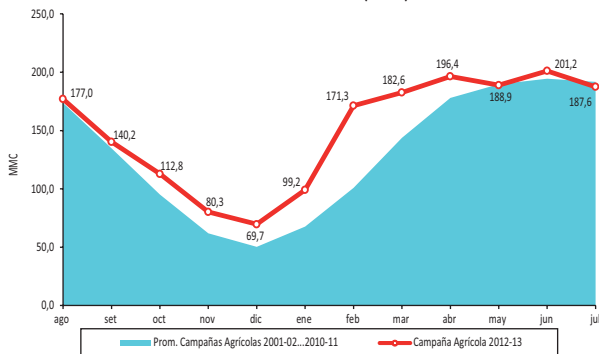
G.83 VOLUMEN DE AGUA ALMACENADA PROMEDIO MENSUAL EN EL RESERVOIRIO SAN LORENZO (PIURA)
