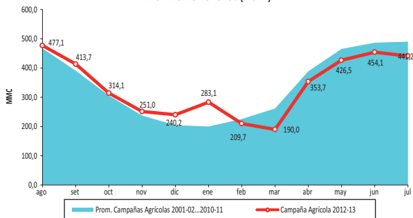
G.84 VOLÚMEN DE AGUA ALMACENADA PROMEDIO/MES EN EL RESERVOIRIO POECHOS (PIURA)
